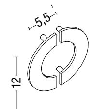
Maniglia Handle Ручка
